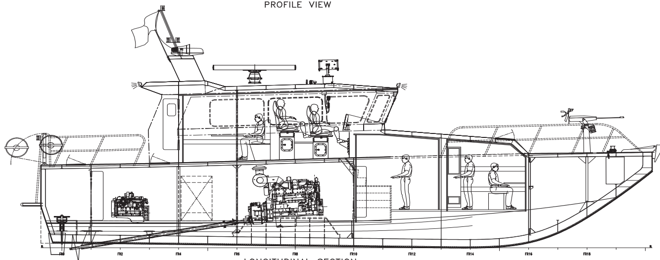
LONGITUDINAL SECTION
